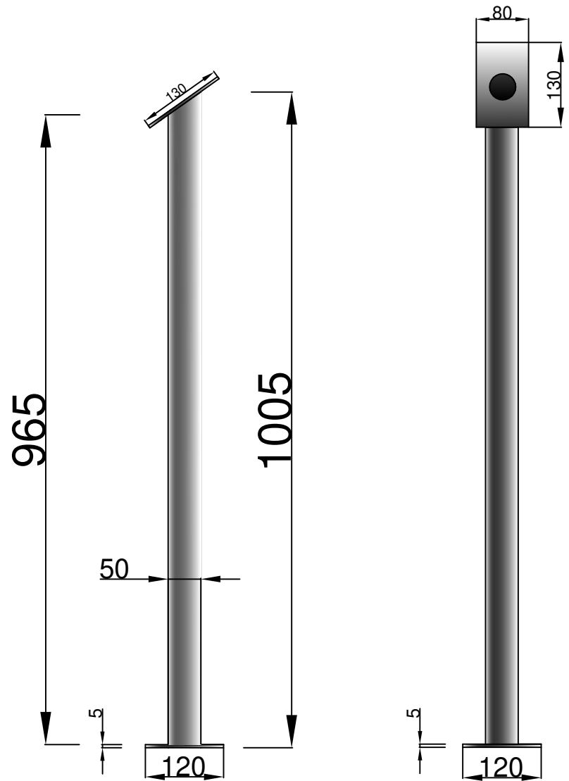
SŁUPEK POD CZYTNIK 130X85 STAL 304 N SZLIF nr katalogowy 10007
